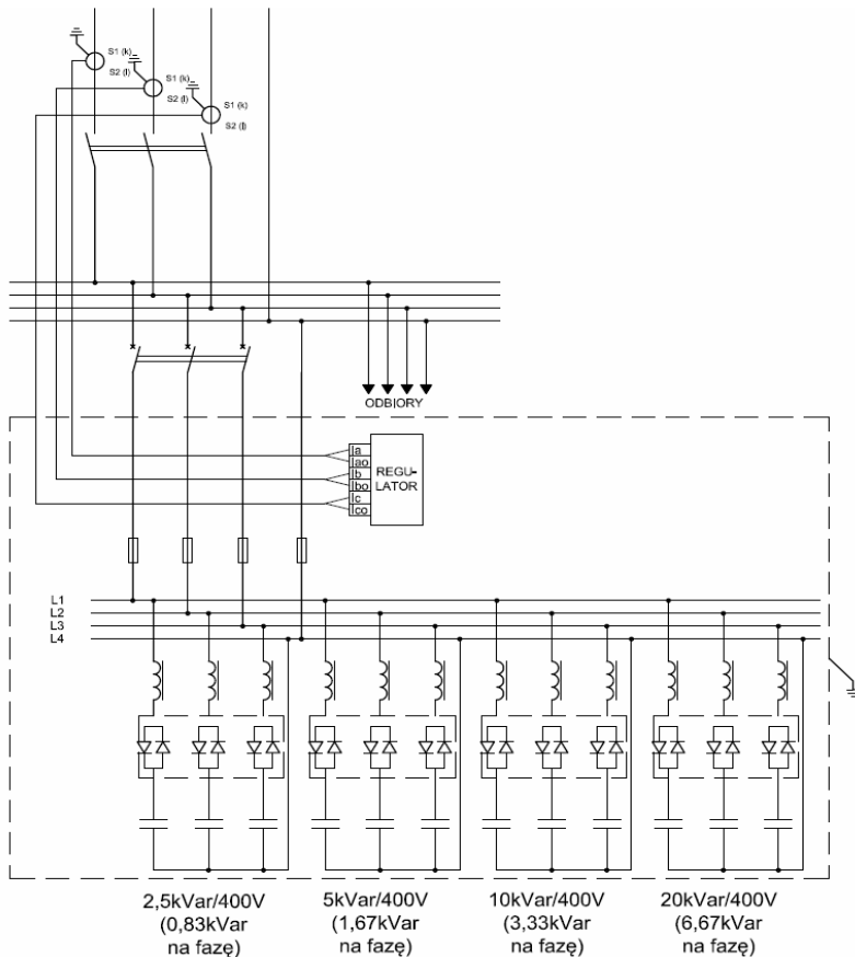
Rys. 1. Schemat podłączenia baterii 37,5/2,5kVAr/400V ze sterowaniem w każdej fazie oddzielnie
